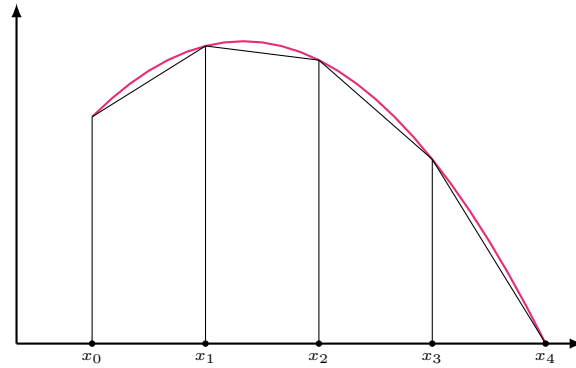
Méthode des trapèzes (ici n = 4 )
